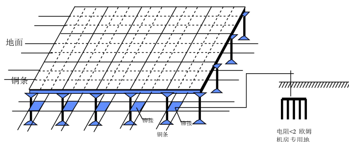
地面架空静电地板示意图
